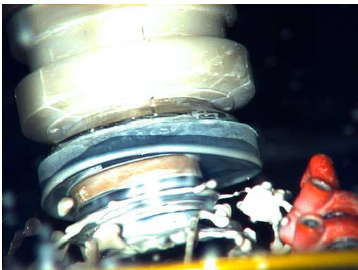
Abbildung 4: Ein an einer frei beweglichen Pinole befestigtes rotierendes Polierpad muss über dem ebenfalls rotierenden Träger, auf dem das Gleitsichtbrillenglas befestigt ist, so gesteuert werden, dass ein gleichmäßiger Abtrag entsteht, durch den das Brillenglas erst durchsichtig wird
