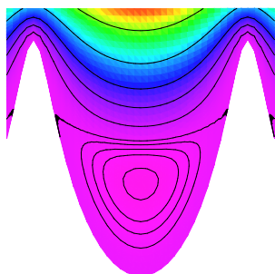
Abbildung 3: Die Flüssigkeit fließt längs der Linien (Stromlinien). Unten entsteht ein Wirbel, der vom Hauptstrom des Flüssigkeitsfilms getrennt ist (aus einer Computersimulation)
