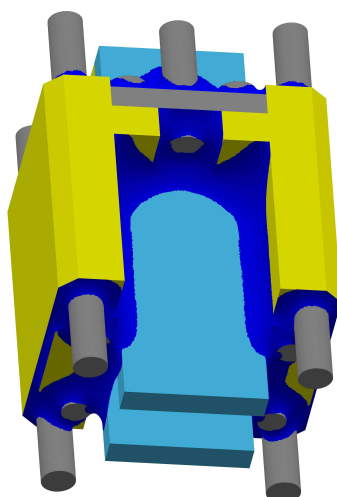
Abbildung 6: Flüssigkeitsbenetzung einer Apparatur bei Flüssigkeitsaustritt unter Schwerelosigkeitsbedingungen. Die Flüssigkeit (dunkelblau) „kriecht“ in alle Ecken und Kanten der Apparatur (Computersimulation)
